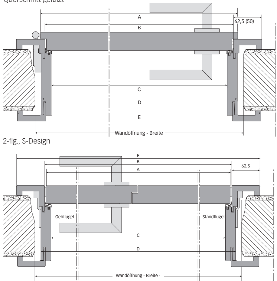
Querschnitt gefälzt
