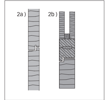
2b ) Türblatt mit Blockrahmen und Füllung
