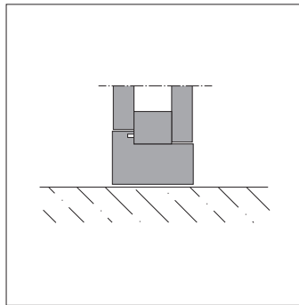
1 ) Boden- / Deckenprofil
