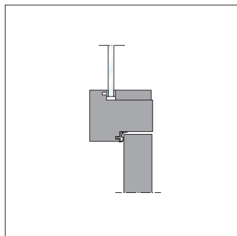
7 ) Kämpfer für Oberlicht in Kombination mit einer Tür
