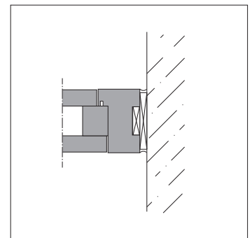
9) Wandanschlussprofil
