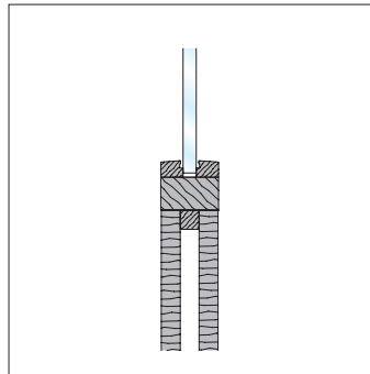
5) Oberlicht in Kombination mit einer Füllung
