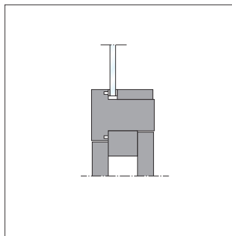
5) Kämpfer für Oberlicht in Kombination mit einer Füllung
