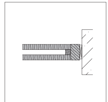
9) Wandanschluss
