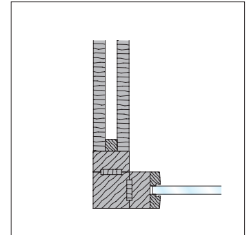
4) Eckprofil
