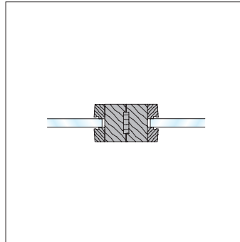
3) Festverglasung an Festverglasung
