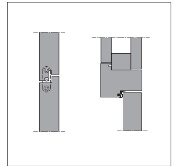
2 ) Türblatt mit Blende wahlweise mit oder ohne Kämpfer
