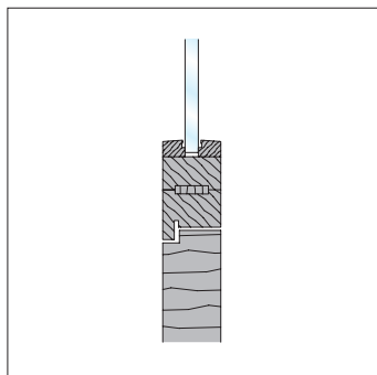
7 ) Festverglasung in Kombination mit einer Tür
