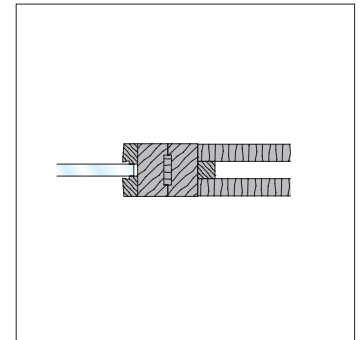
6 ) Festverglasung an Füllung
