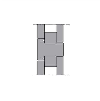
8) Kämpfer für Füllung an Füllung
