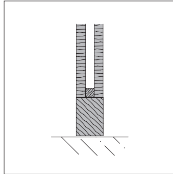
1 ) Boden- / Deckenprofil
