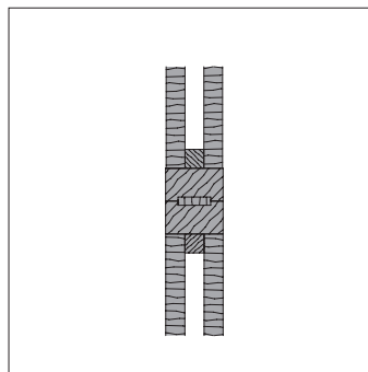
8) Füllung an Füllung
