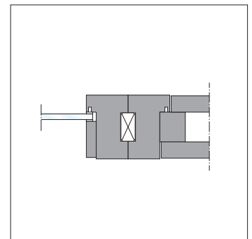
6 ) Glas an Füllung
